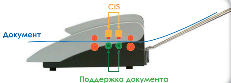
Сканер KIP 720 имеет систему поддержки для улучшения надежности протяжки оригиналов
