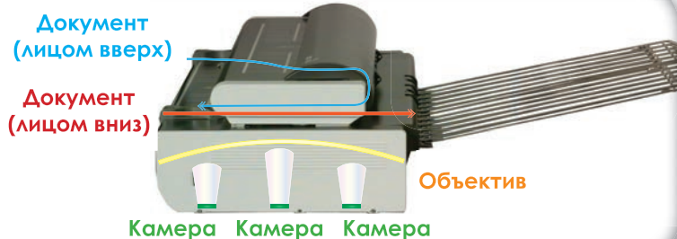
Три независимые CCD-матрицы в сочетании с улучшенной лазерной системой юстировки и автоматической калибровкой обеспечивают наивысший уровень качества сканирования
